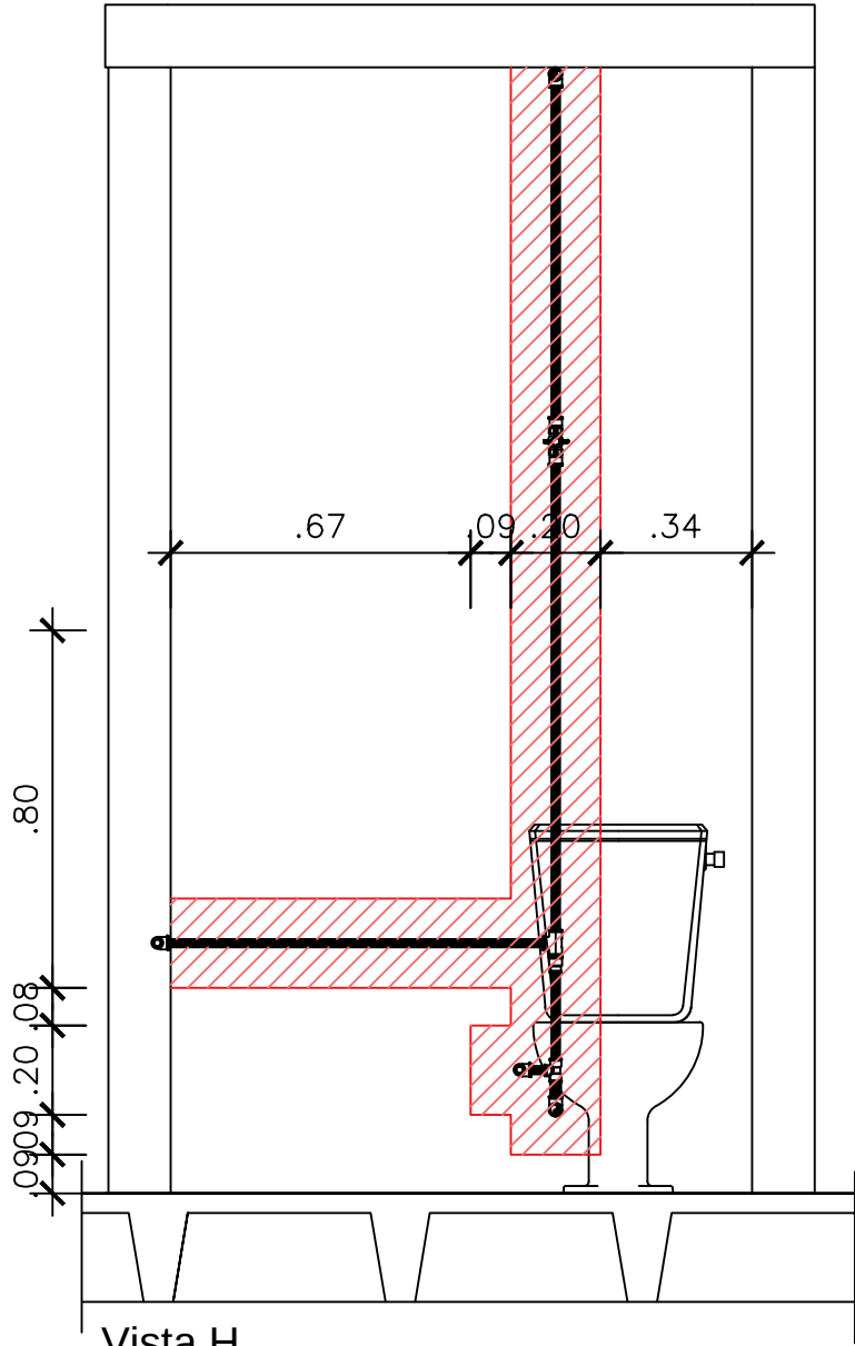
Vista H ESCALA 1/25
