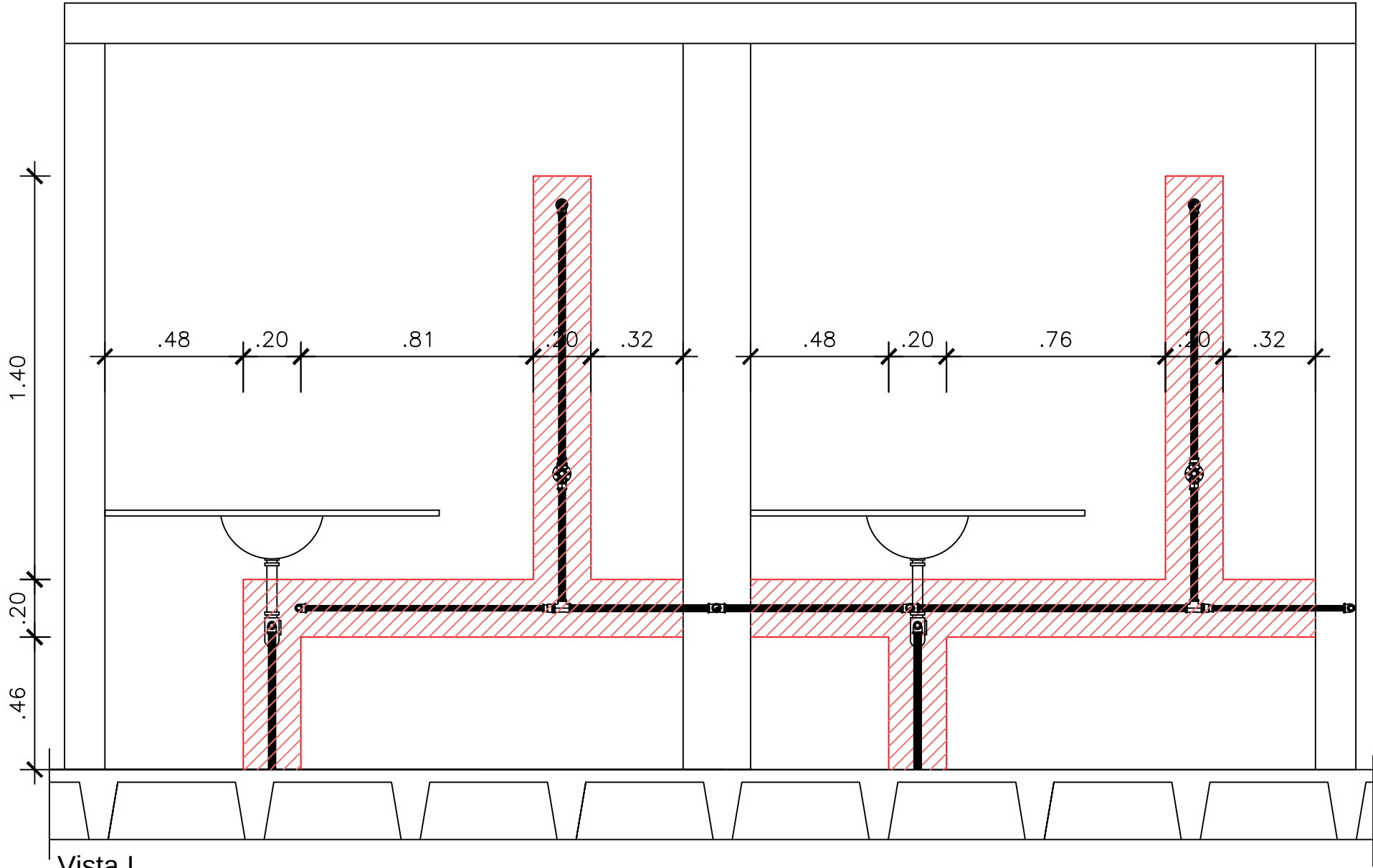
Vista I ESCALA 1/25
